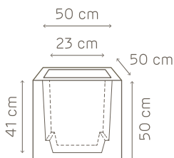
art. 2585 pot gloss cm.50
